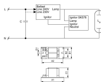
Scheda tecnica Lampada HID Philips BSN 400 K407-ITS 230/240V 50Hz BC3-166
